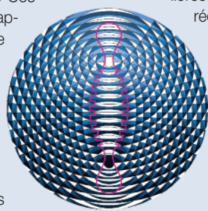
Rayonnement géométrique
